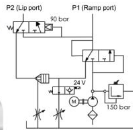
DOCK LEVELER SWING TYPE MENTEŞELİ RAMPA
